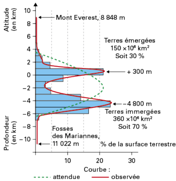
Figure 2. Distribution des altitudes sur la croûte terrestre
