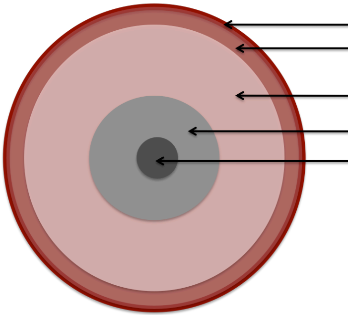
Figure 1. Structure interne du globe terrestre
